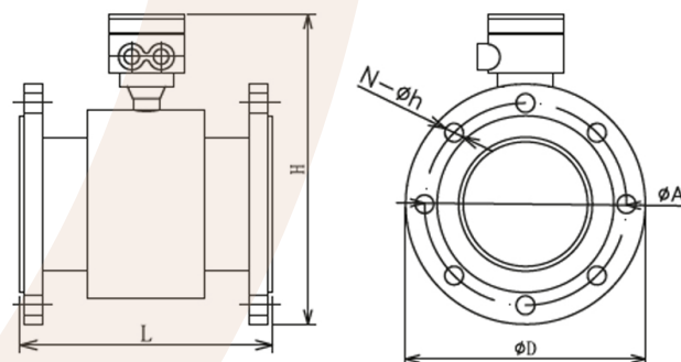
DN15-DN600 Электромагнитный расходомер в разнесенном исполнении со стандартом фланца DIN
