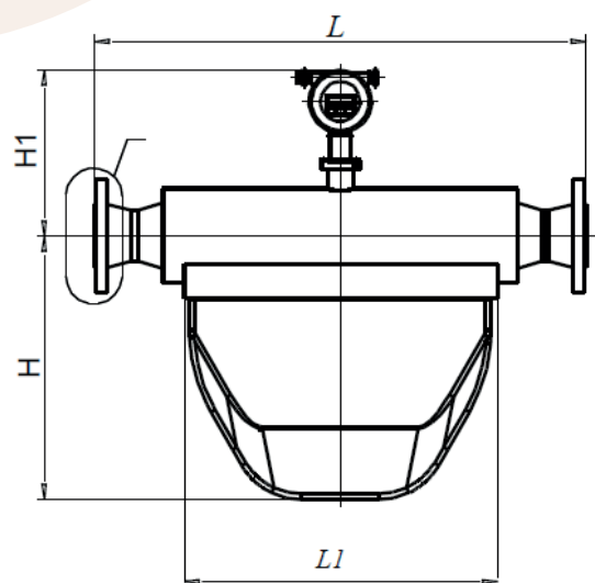
Интегральное исполнение - рис. А.2.1 (серия М)
